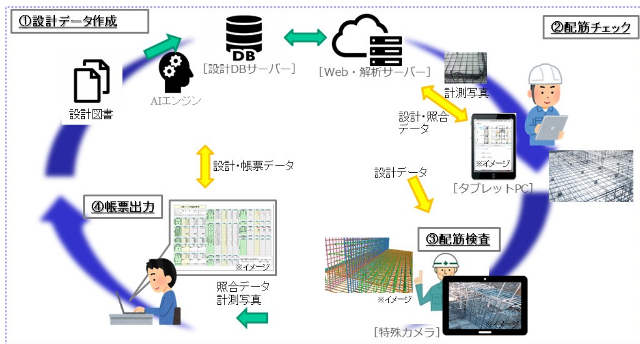
「配筋検査システム」の実装イメージ
