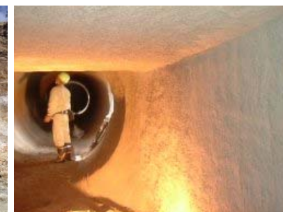
コークス炉の出口煙道耐火工事 (耐火工事)
